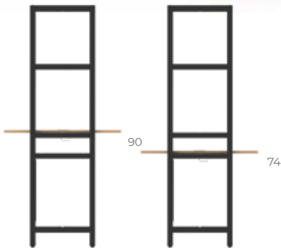
SMART L 208 x 90 x 186
